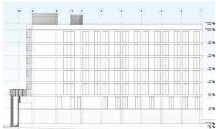
Right elevation
